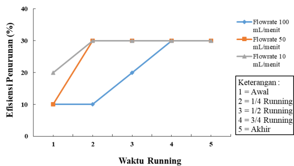
Gambar 2. Pengaruh Flowrate terhadap Efisiensi Penurunan pH
