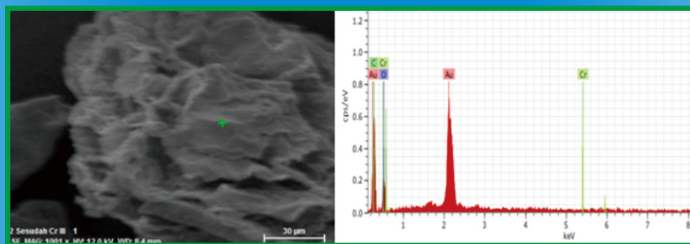
FE-SEM dan Spektrum EDX dari Biji Buah Bisbul Setelah Menyerap Ion Logam Cr(III)
